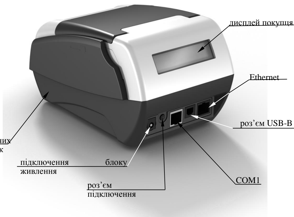
Рис. 2 Задня панель
